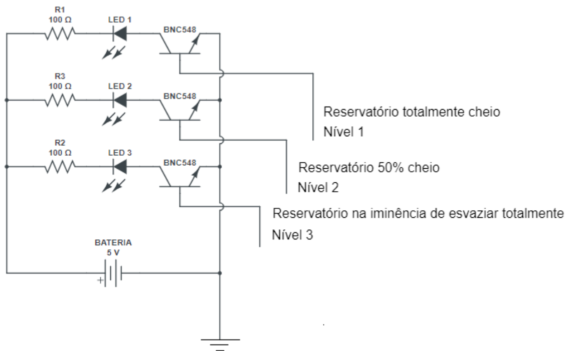
Figura 1 - Diagrama de circuito do medidor composto por três níveis
